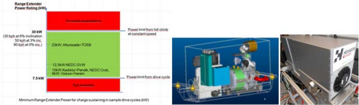
Şekil 5. Menzil Uzatici Boyutlandırılması ve Menzil Uzatici Sistem Tasarımı
