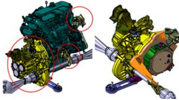
Şekil 6. Mevcut Dizel Motor Bağlantısı ve Elektrik Motoru Adaptasyonu
