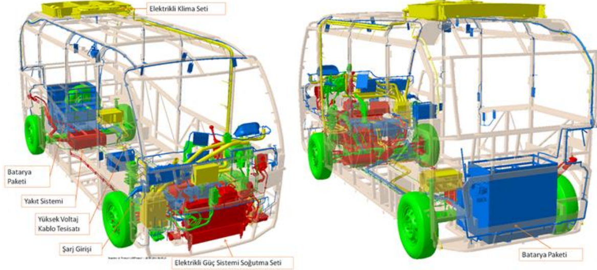
Şekil 3. Menzil Uzatıcı Elektrikli Minibüs Paketleme Görüntüsü
