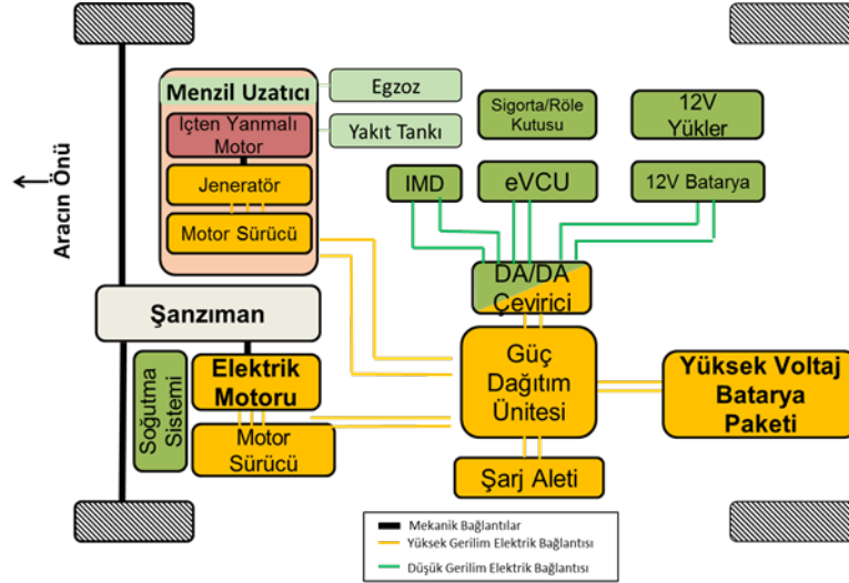
Şekil 2. Menzil Uzaticılı Elektrikli Minibüs Blok Şeması(REEV: Range Extended Electric Vehicle)
