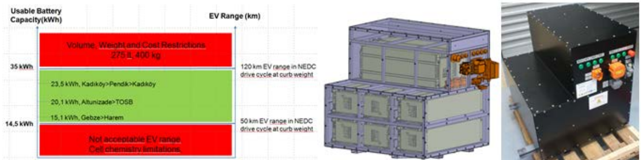
Şekil 4. Batarya Boyutlandırılması ve Batarya Paketi Tasarımı
