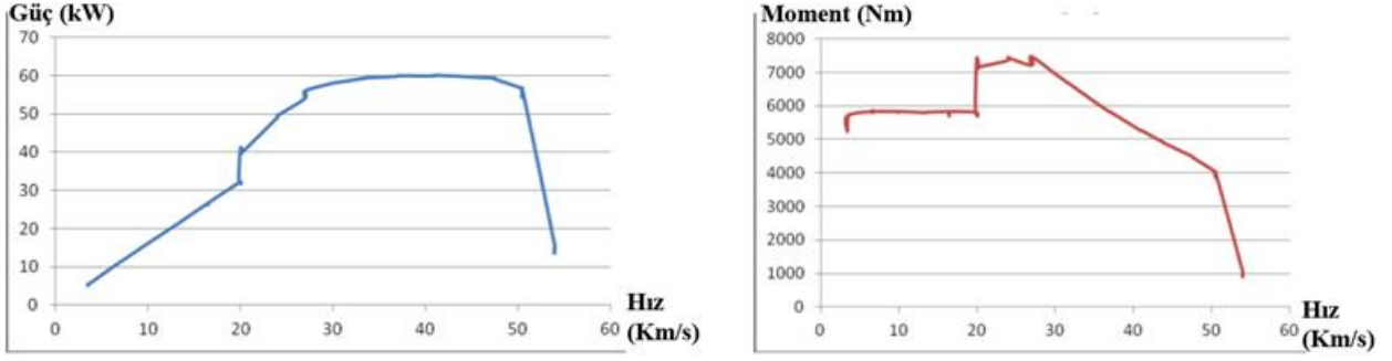
Şekil 10. Şasi Dinamometre Performans Test Sonuçları (Sol: Güç Eğrisi; Sağ: Tork Eğrisi)
