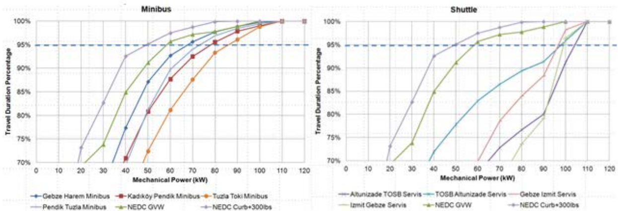
Şekil 1. Minibüs ve Personel Servis Hatları Performans Gereksinimleri
